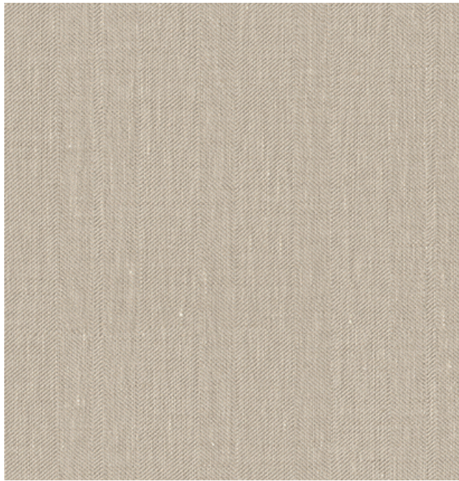
008 Ion
