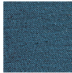
005 Doppler
