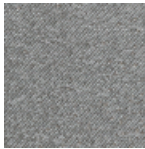
004 Flux
