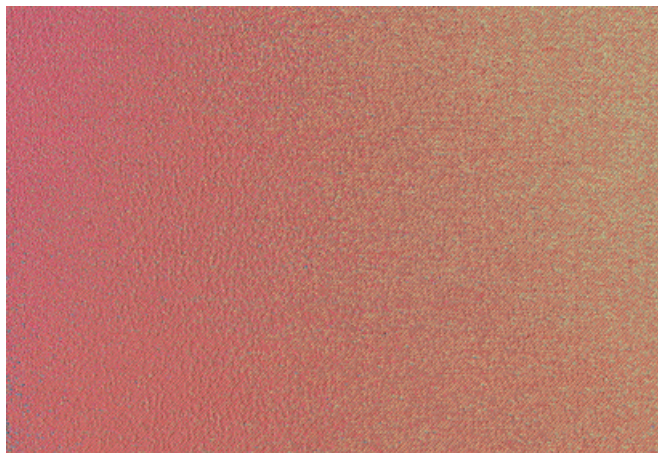
001 Quantum
