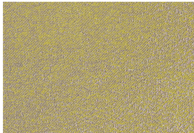
003 Proton
