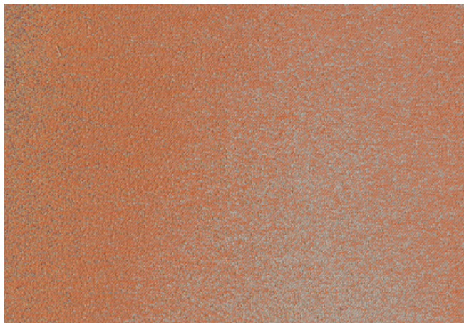
002 Pulsar
