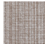
007 Hubble
